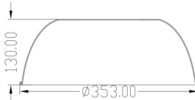
90° AL Reflector Size
